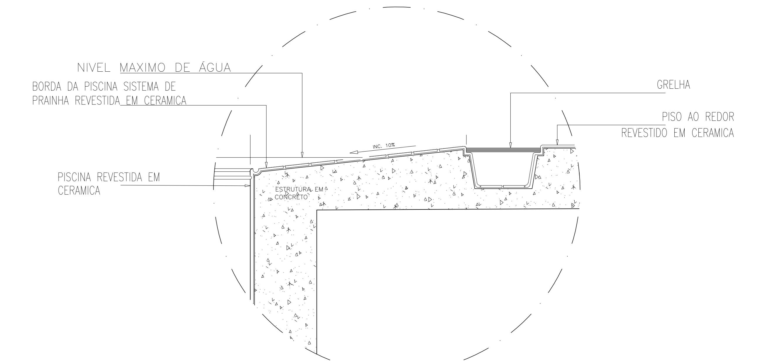
DETALHE DE BORDA
