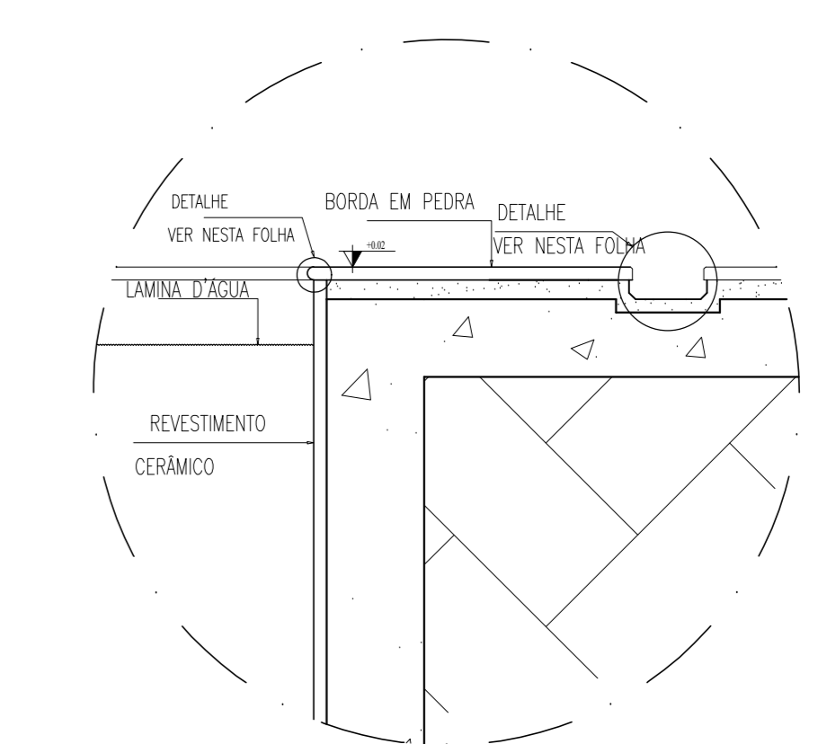
DETALHE-BORDA DA PISCINA
