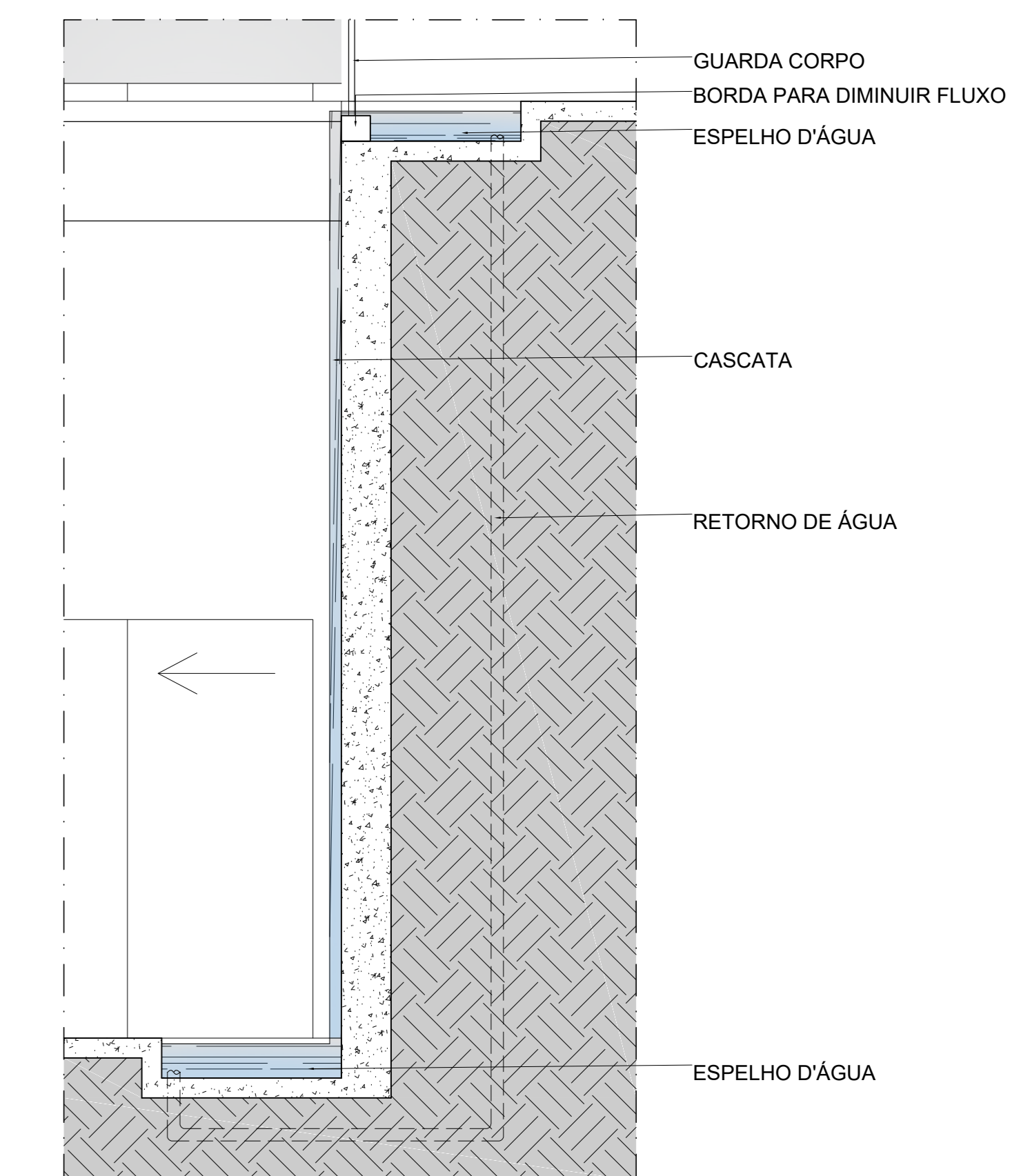
DETALHE CASCATA ESCALA 1:25
