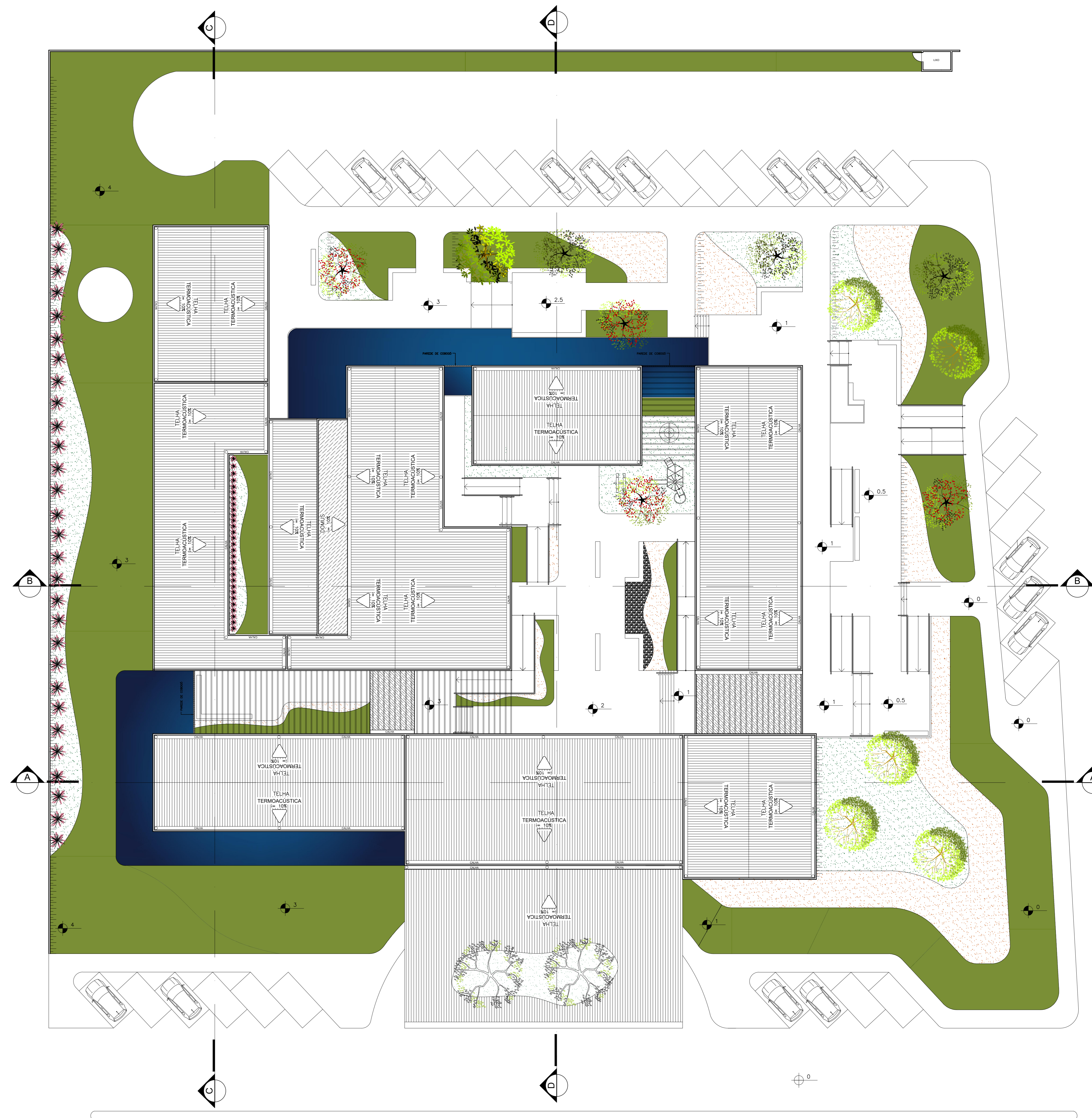
2 COBERTURA ESCALA 1:200
