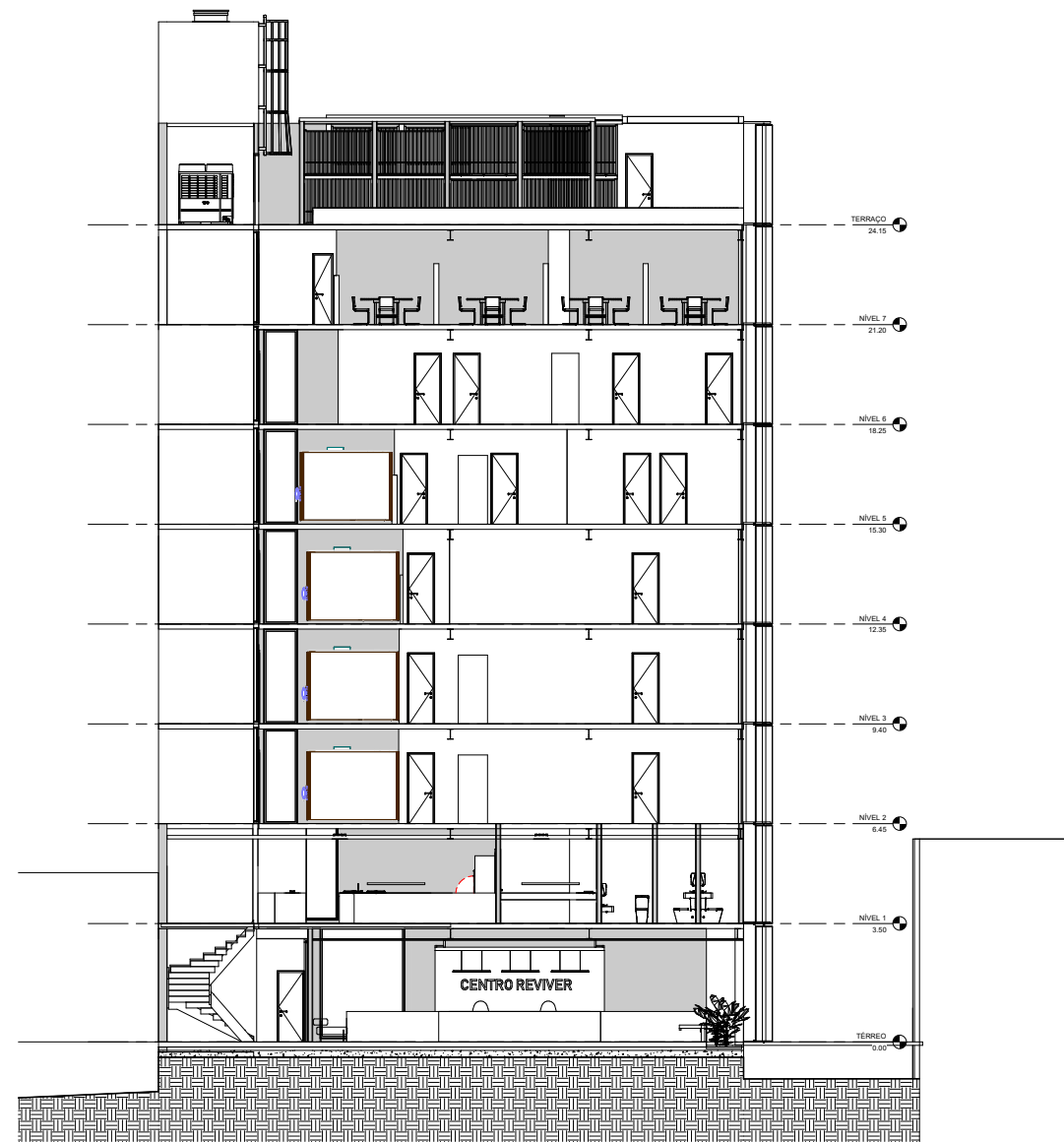
① CORTE AA 1:50
