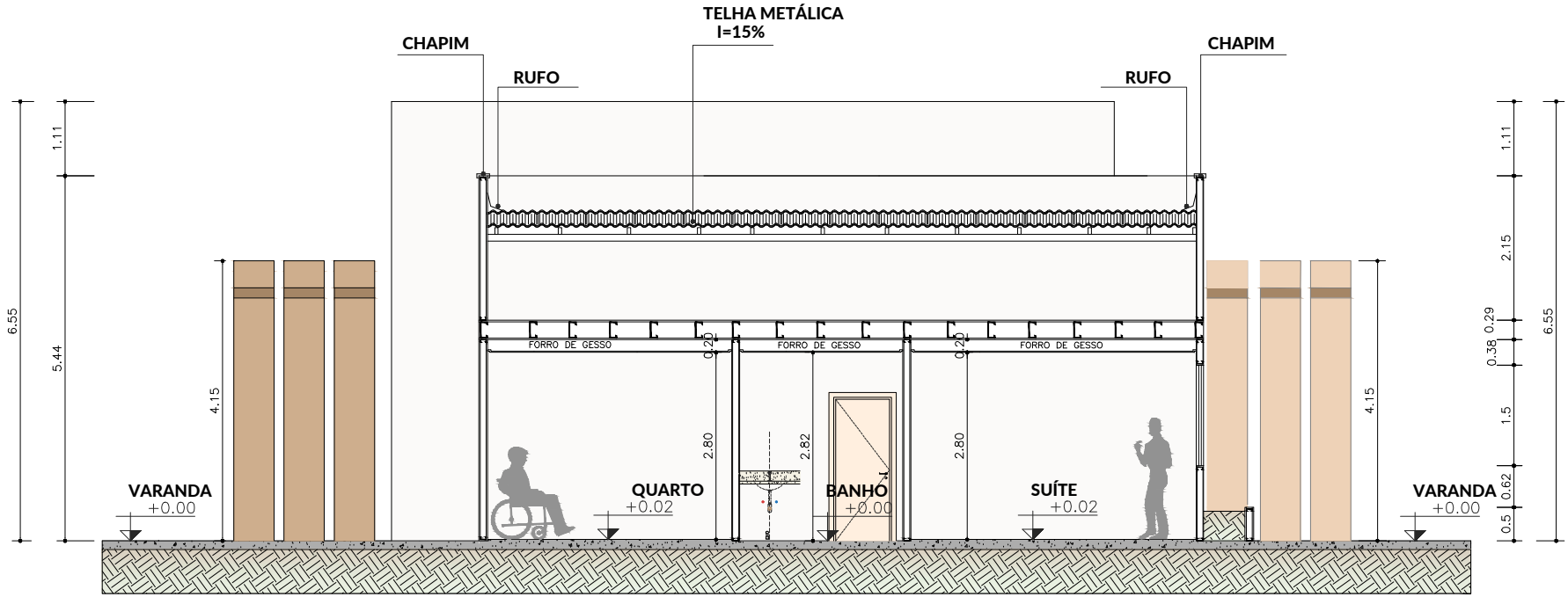
CORTE BB TIPOLOGIA 1 E 2 ESC. 1:100
