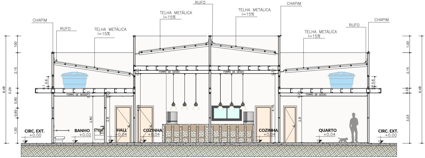
CORTE AA TIPOLOGIA 1 E 2 ESC. 1:100
